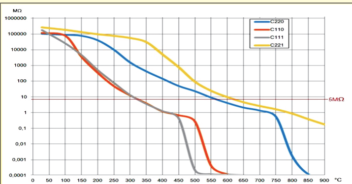
Curvas de variación de resistividad de aislamiento de bloques de terminales en función de su temperatura llevadas a cabo en distintos tipos de cerámica, (C110, C111, C220, C221) en un grosor de 2 mm. El valor 5MΩ es el límite normativo.
